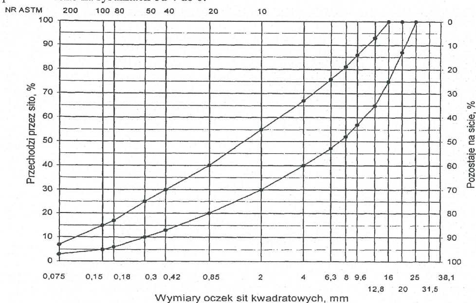
Rys. 4. Krzywe graniczne uziarnienia mieszanki mineralnej BA od 0 do 20 mm do warstwy wiążącej nawierzchni drogi o obciążeniu ruchem KR1-2
