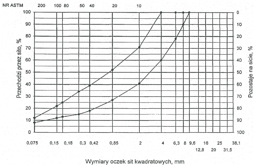
Rys. 3. Krzywe graniczne uziarnienia mieszanki mineralnej BA od 0 do 8mm, od 0 do 6,3 mm do warstwy ścieralnej nawierzchni drogi o obciążeniu ruchem nawierzchni drogi o obciążeniu ruchem KR 1-2
