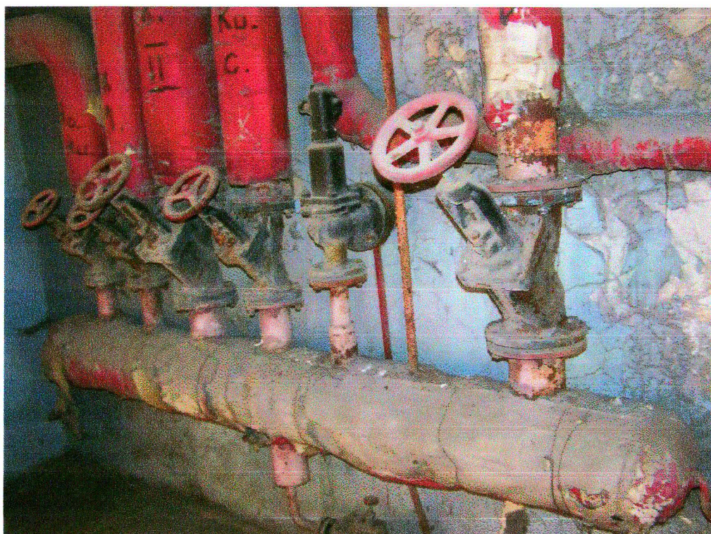
Rury instalacji technologicznej-rozdzielacz
