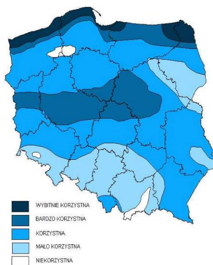
Rysunek 7. Strefy energetyczne wiatru na obszarze Polski
