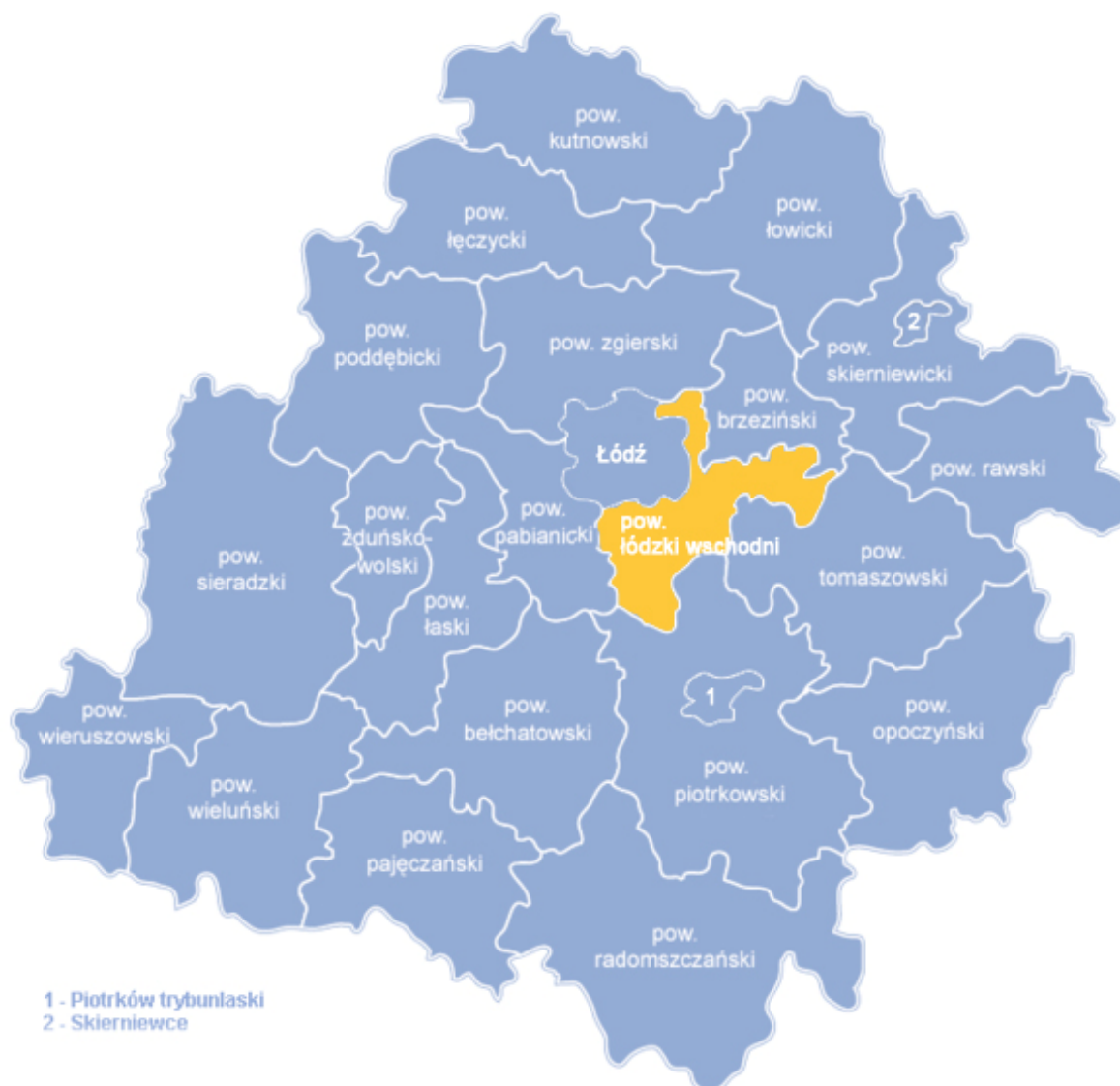
Rysunek 2. Położenie Powiatu Łódzkiego Wschodniego na obszarze województwa łódzkiego
